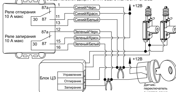
Схема подключения к блоку ЦЗ с управлением импульсами положительной полярности и есть мастер-переключатель в водительской двери : CHRYSLER, MERCURY SABLE
