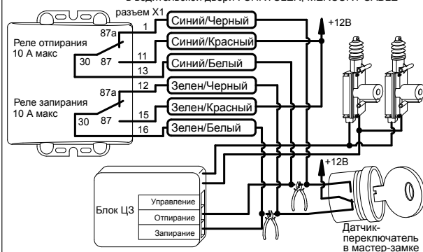
Схема подключения к блоку ЦЗ с управлением импульсами положительной полярности и есть мастер-переключатель в водительской двери : CHRYSLER, MERCURY SABLE
