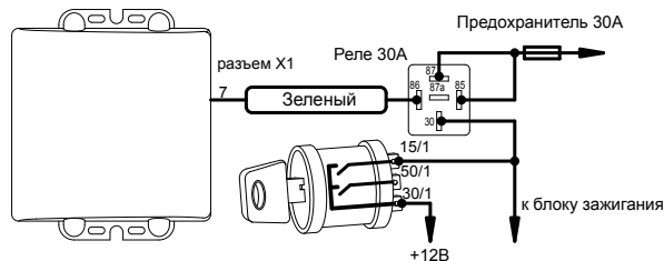
Рис. 13 Пример схемы для реализации функции поддержки зажигания с помощью Таймерного канала №1 (при программировании назначить таймерный канал для выполнения этой функции)
