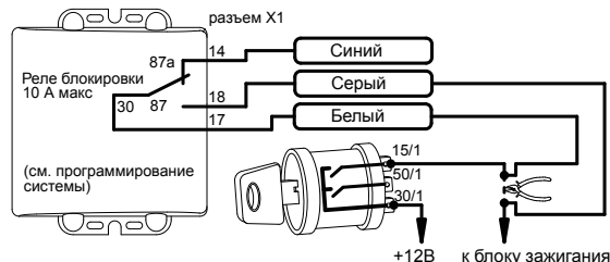
Пример схемы блокировки нормально разомкнутым реле (перепрограммировать тип контактов НР)
