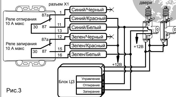
Схема подключения к блоку ЦЗ с управлением импульсами положительной полярности и есть мастер-переключатель в водительской двери : CHRYSLER, MERCURY SABLE
