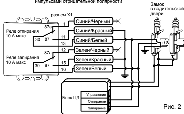
Схема подключения к блоку ЦЗ с управлением импульсами отрицательной полярности
