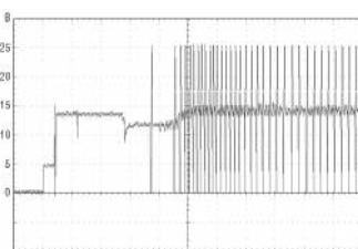
Сигнал форсунок
