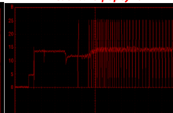
Сигнал с форсунок
