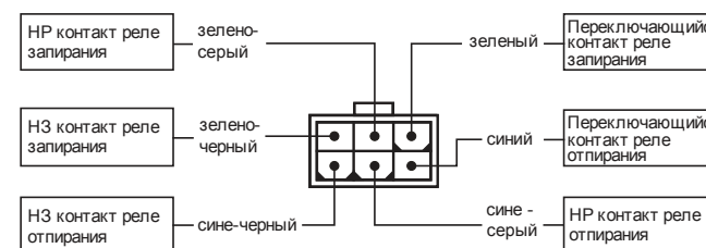
Назначение контактов разъема «Х2»:
