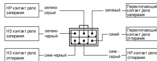
Назначение контактов разъема «Х2»
