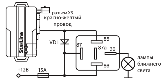
Схема реализации функции «световая дорожка»
