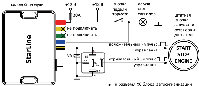
Схема 1: силовое управление кнопкой «старт-стоп»
